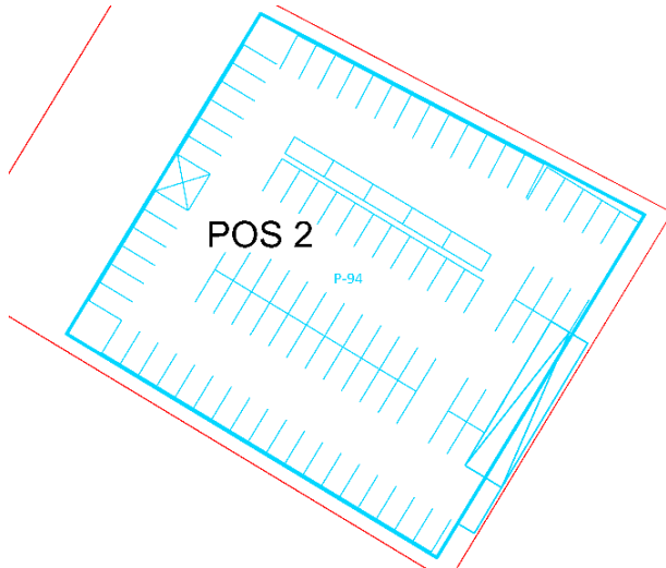
Skeem 4. Pos 2 näitlik maa-aluste parkimiskohtade paiknemine ühel maa-alusel korrusel (94 parkimiskohta). Arvestatud on, et rambi rajamisel väheneb joonisel 4 Pos 2 esitatud maaapealsete parkimiskohtade arv u 11 võrra (41-lt 30-le).
