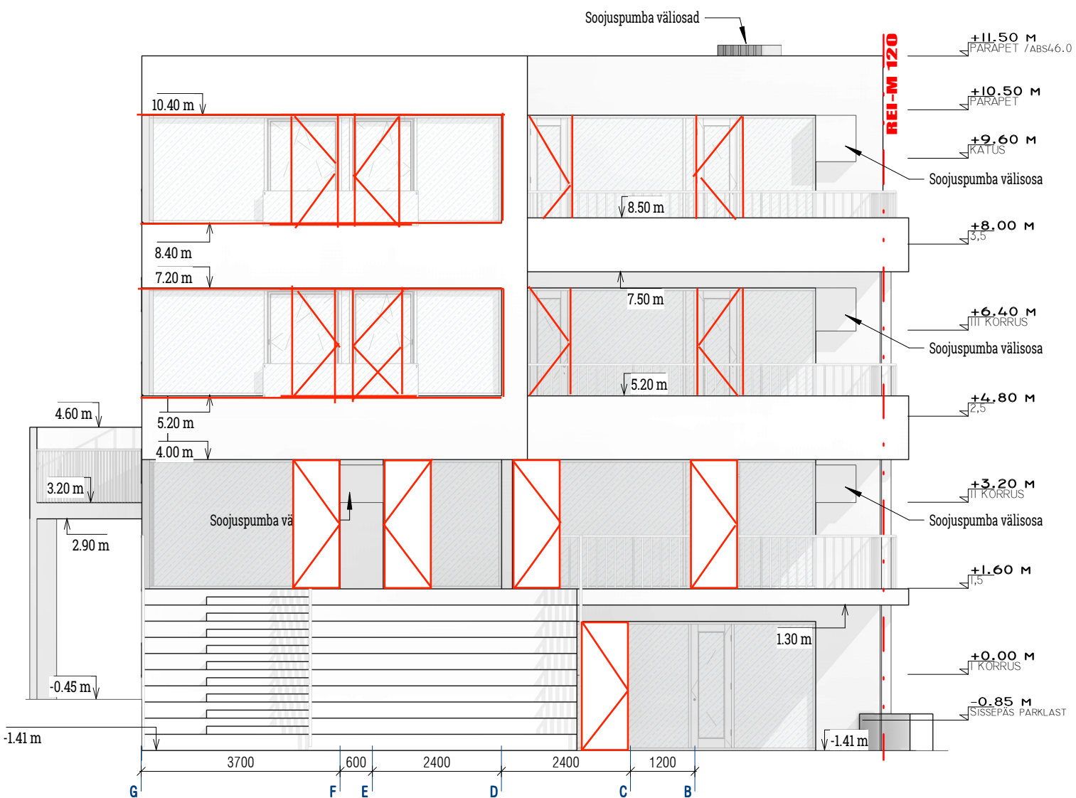
HOOVIMAJA/ VADE PÕHJAST 1 : 100
