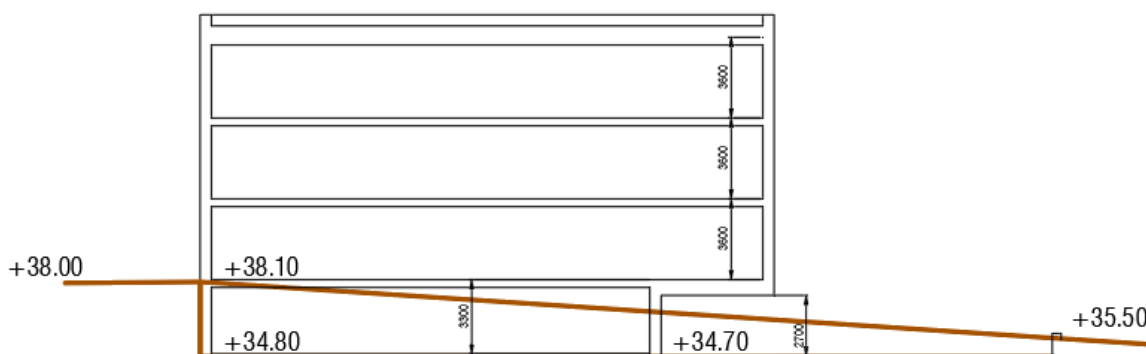
Skeem 2. Näide hoone 0.00 kõrguse kujunemisest reljeefsel pinnal.
