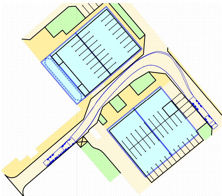
Pöörderaadiuste skeem.
