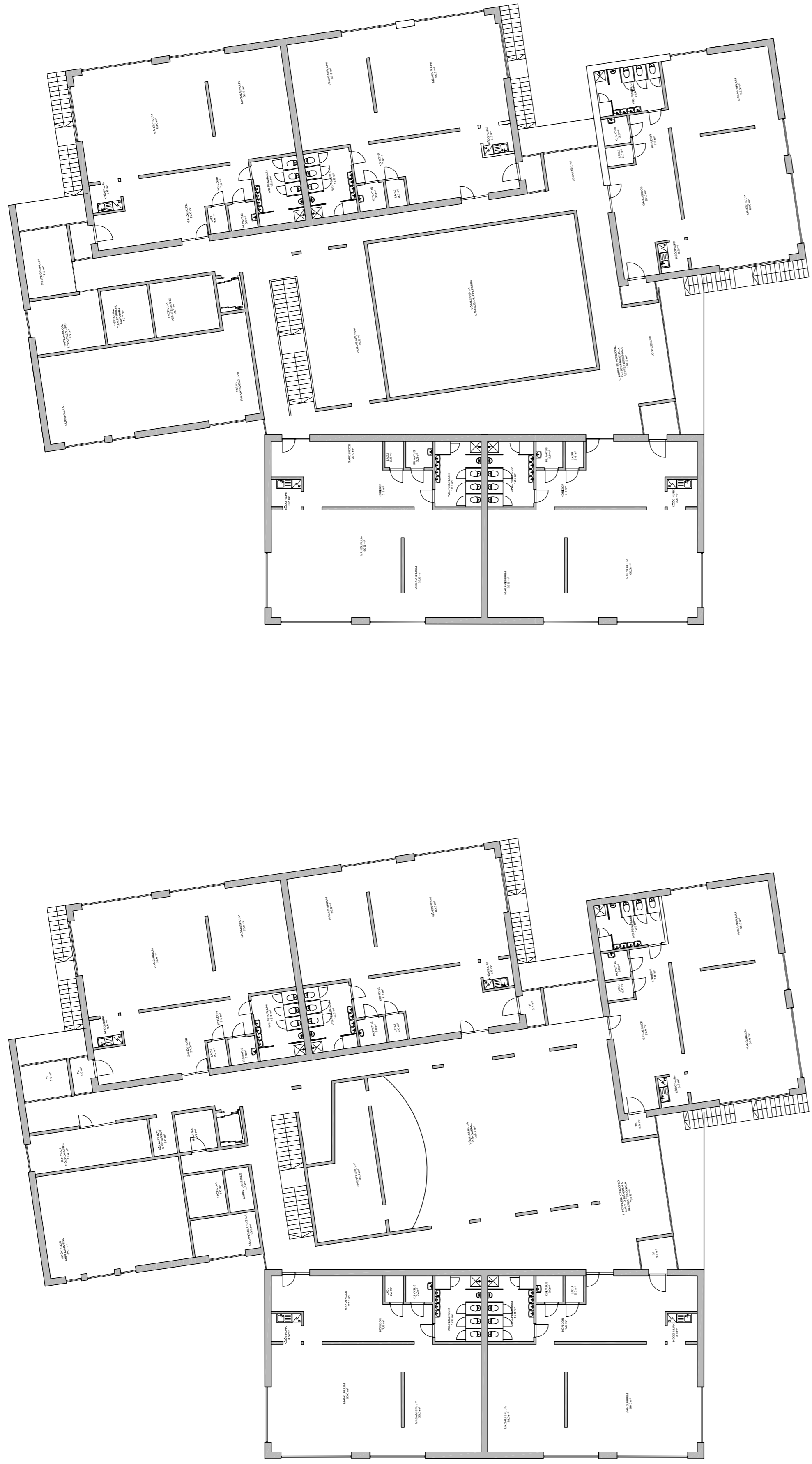
1. KORRUSE PLAAN
