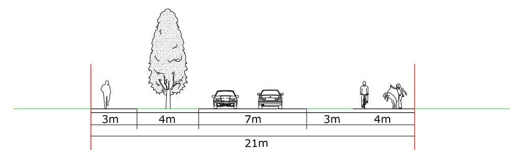
Lõige A-A
