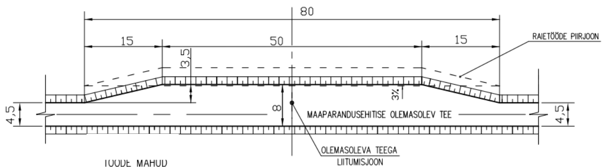
Skeem 3. Möödasõidutasku tööprojekt. (Allikas: Maaparandusrajatiste tüüpjoonised)
