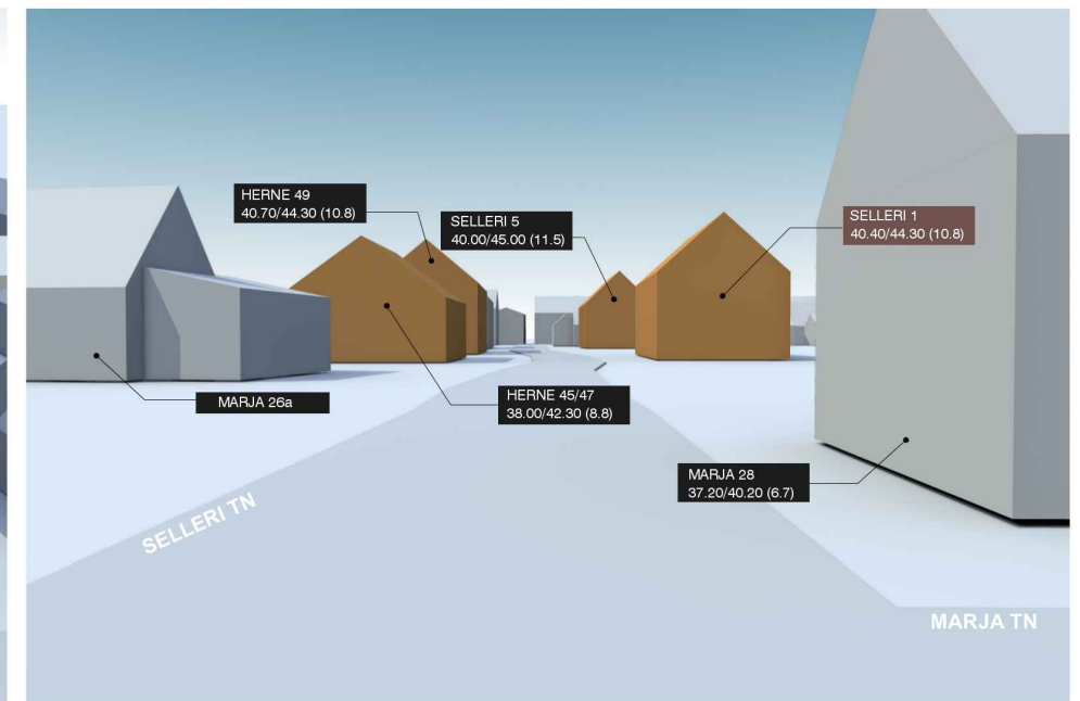
VAADE MARJA TÄNAVALT PIKI SELLERIT 40.70/44.30 (10.8) = Räästa abs. kõrgus/Harja abs. kõrgus (harja kõrgus maapinnast) arhitektuuriklubi oü
