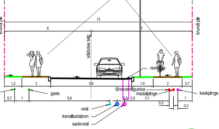
PLANEERITUD TÄNAVA LÕIGE 1-1
