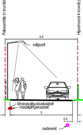
PLANEERITUD TÄNAVA LÕIGE 1-1
