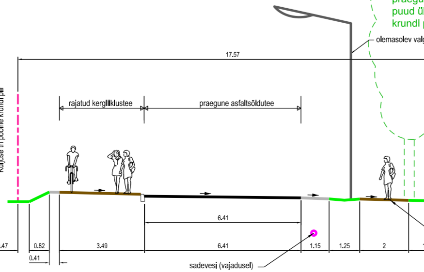
HIPODROOMI TÄNAVA LÕIGE 2-2
