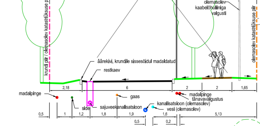
HIPODROOMI TÄNAVA LÕIGE 2-2
