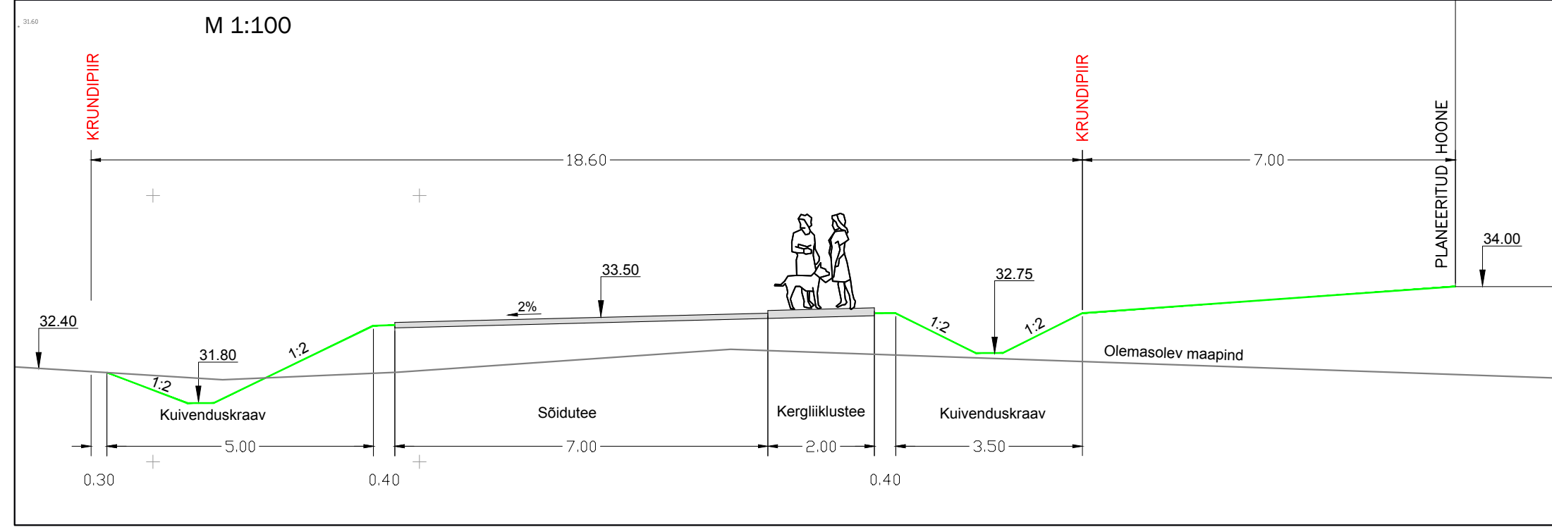
LÕIGE A-A (RANNA PST TEEKORIDOR)
