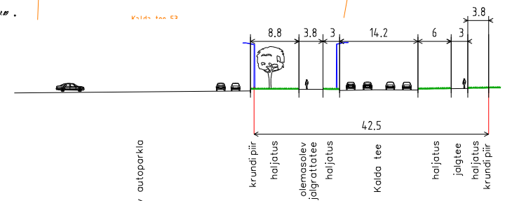
LOIGE 1-1 täna ristprofiil
