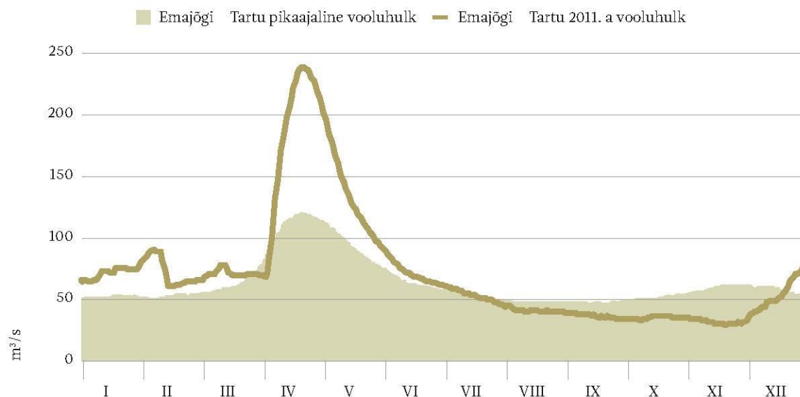
Joonis 4.2. Emajõe pikaajaline keskmine vooluhulk ja 2011. aasta vooluhulk Tartu hüdromeetrijaama andmetel 10 .
