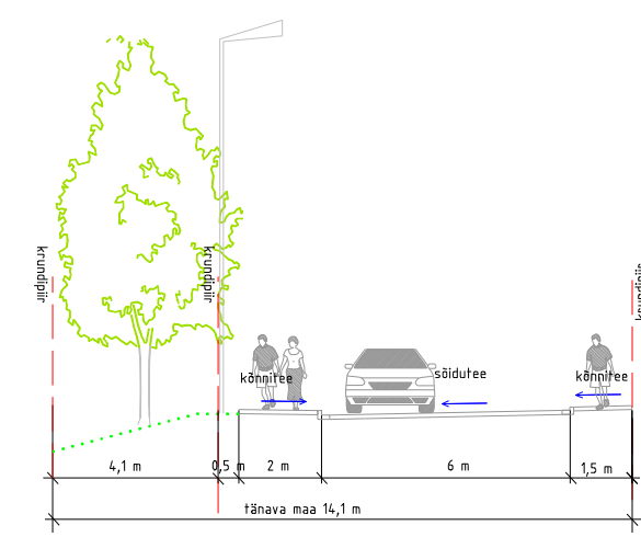
LÕIGE F-F' Kvissentali põik tn
