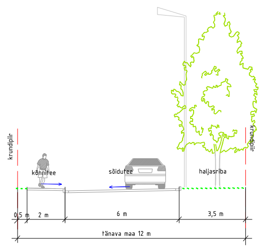
LÕIGE D-D' Tupiktänav
