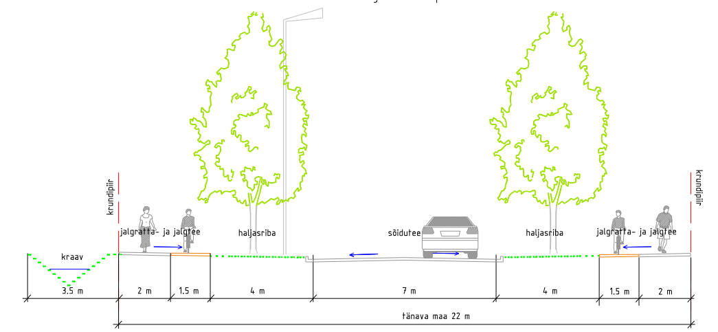
LÕIGE C-C' Ujula tn pikendus
