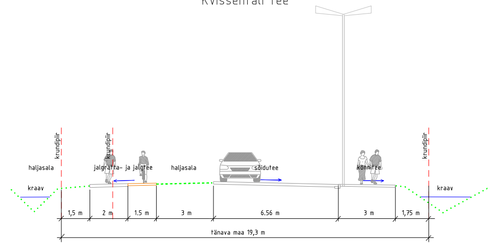
LÕIGE B-B' Kvissentali tee
