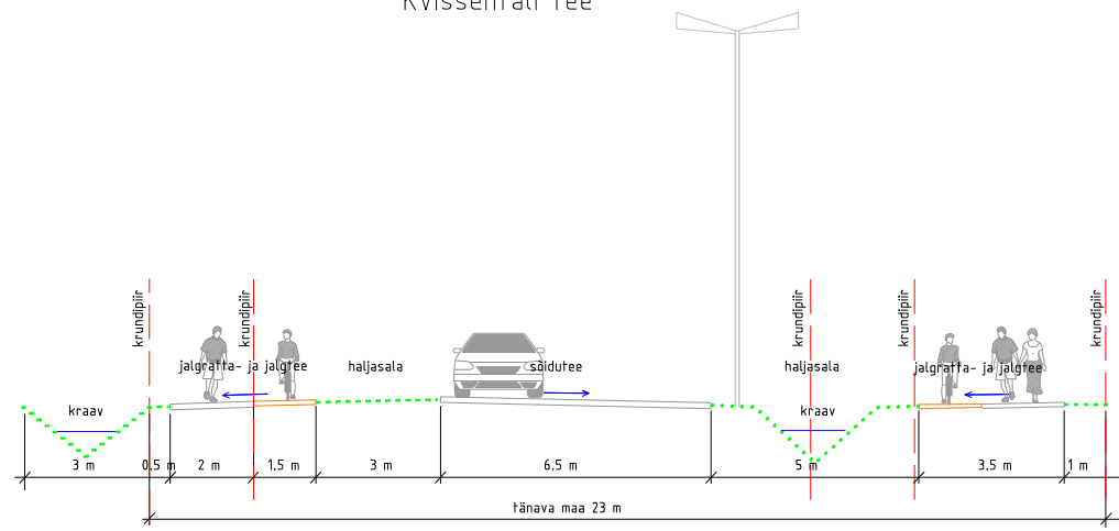
LÕIGE A-A' Kvissentali tee
