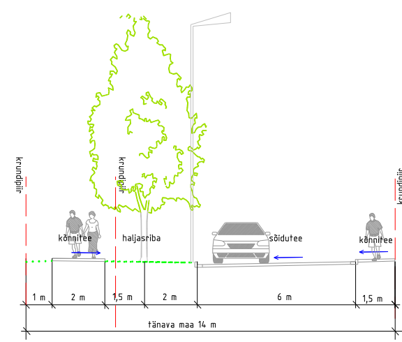
LÕIGE E-E' Kvissentali põik tn
