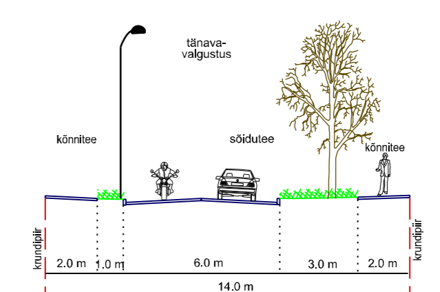
Surnuaia tn ristprofiil 1:200 lõige 1-1
