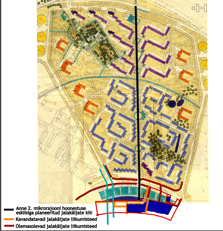
Anne 2. mikrorajooni hoonestuse eskiis aastast 1977
