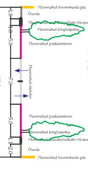
Liige C-C M 1:200
