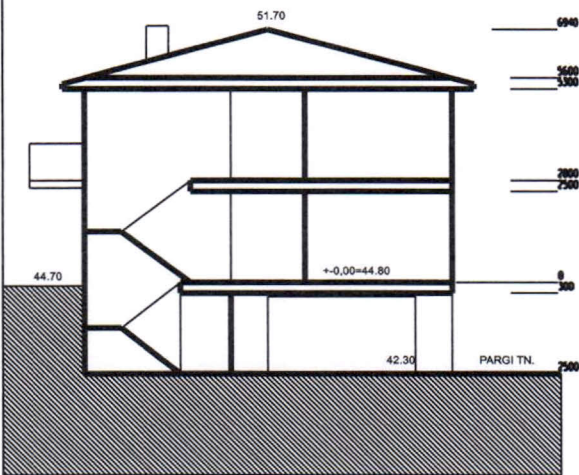
LÕIGE A-A
