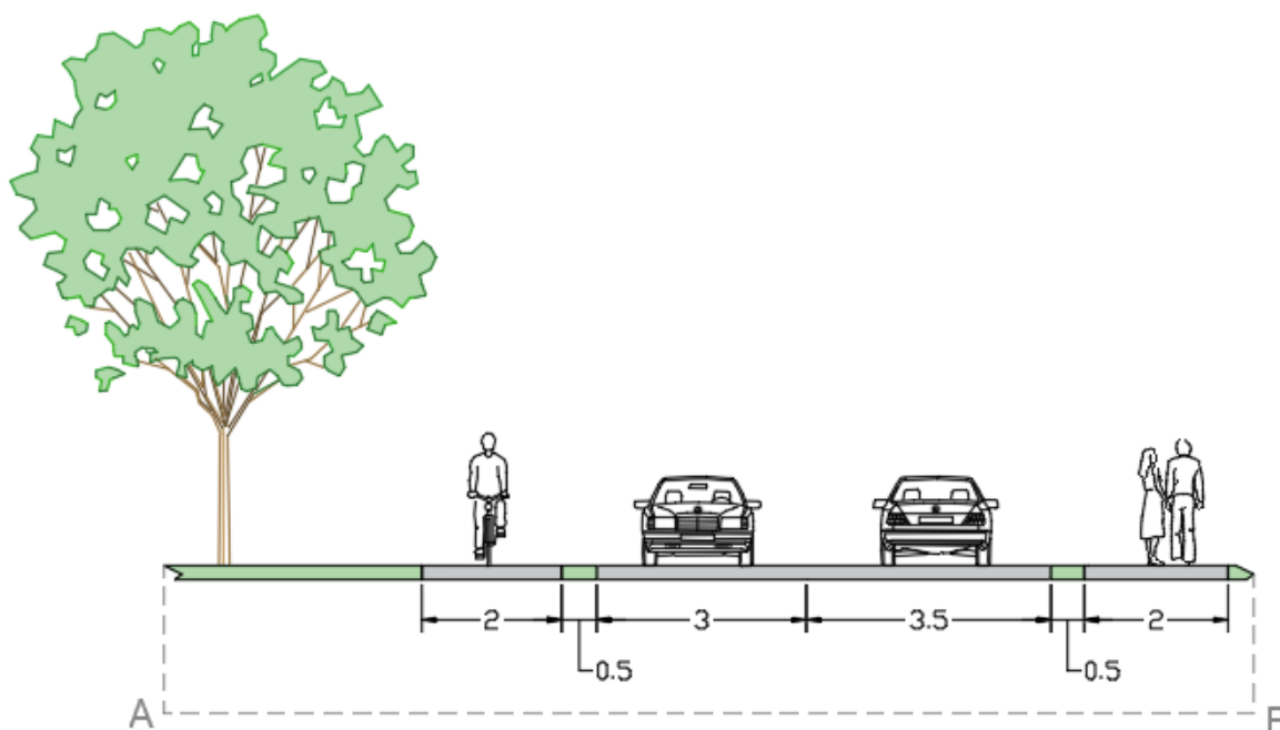
Skeem 2. Lõige A-B planeeritud Lina tänava liikluslahedusest.
