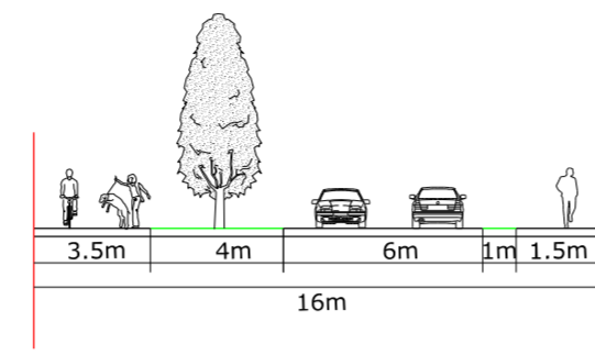
Lõige B-B
