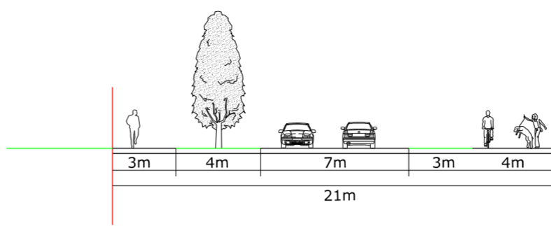
Lõige A-A
