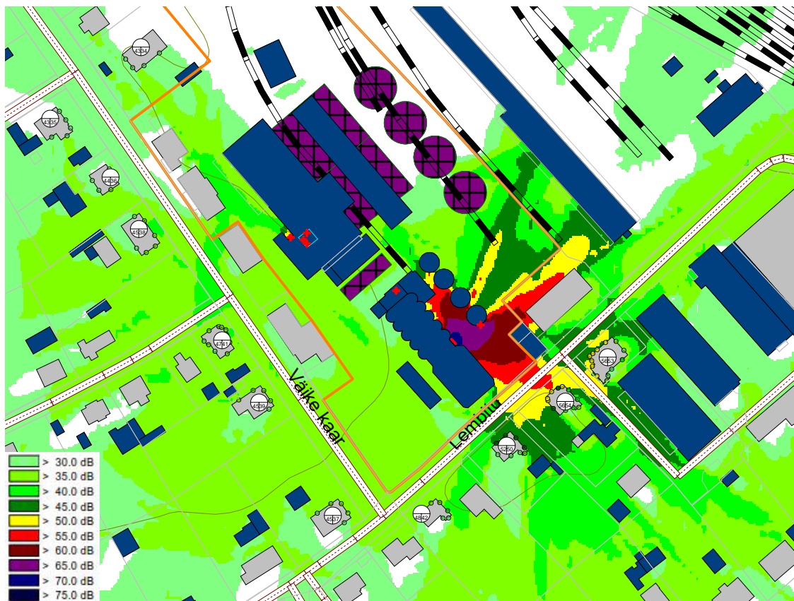
Joonis 9. Seadmete ja elevaatori tööst tingitud hinnatud müratasemed öisel ajavahemikul tootmisüksuse laienduse korral
