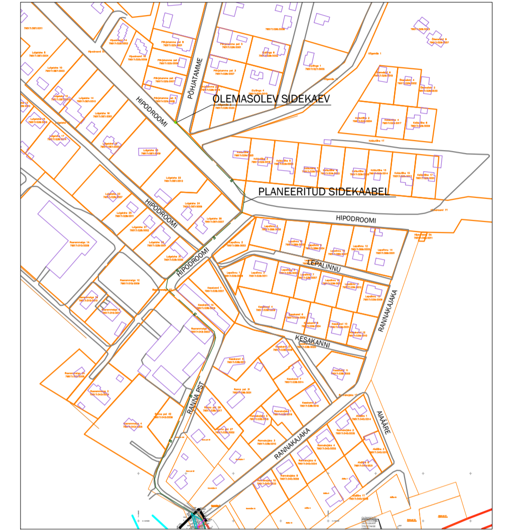
Sidekaabli ühendusskeem Hipodroomi-Põhjatamme nurgal asuva sidekaevuga M 1:4000
