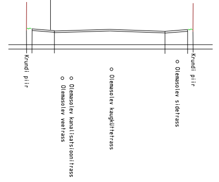
Lõige B-B
