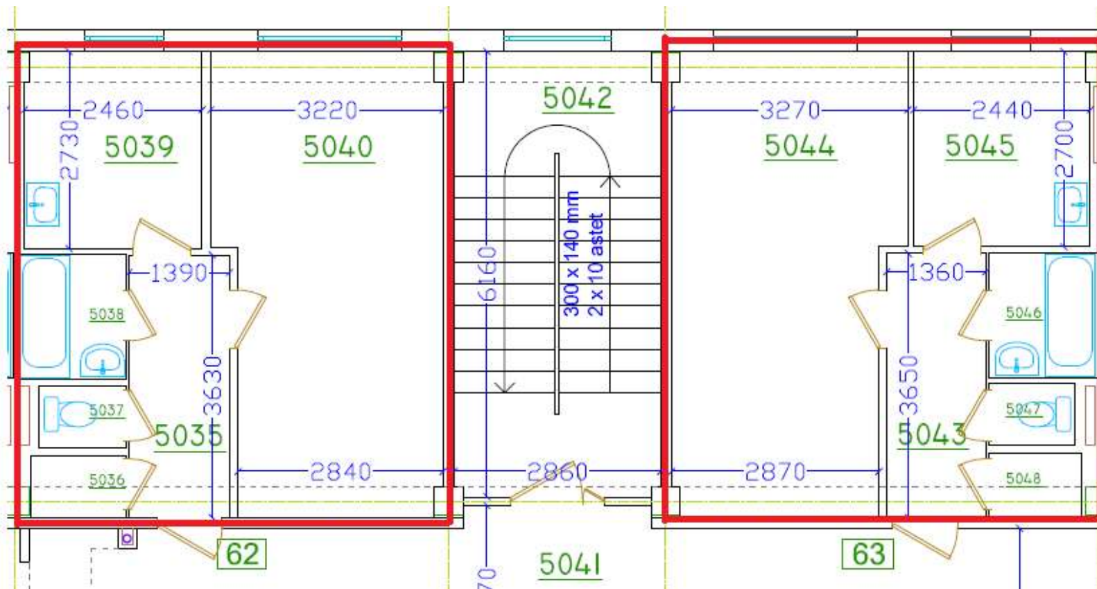
Lisa 1. Korterite Rahu 8 – 62 ja Rahu 8 – 63 plaan.
